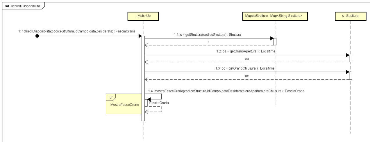
Figura 12: Diagramma di sequenza di Richiedi disponibilit 
